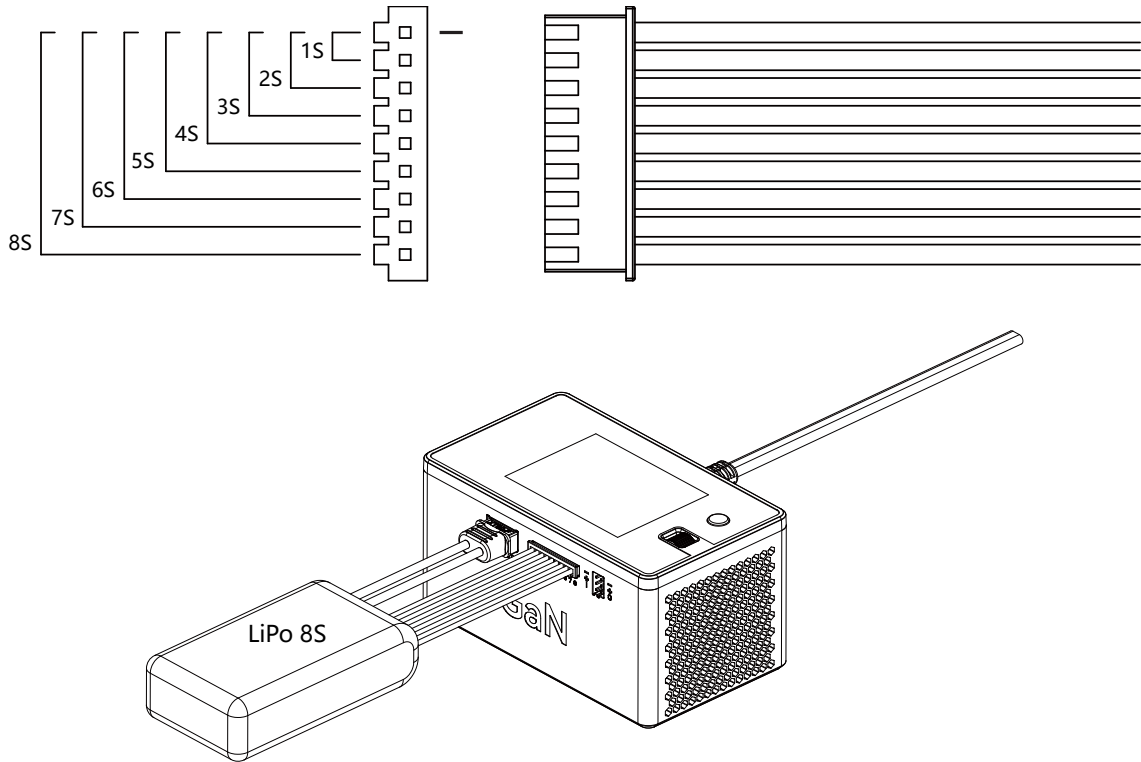
Balanceranschluss für Lithium-Akkus von 1S bis 8S.
