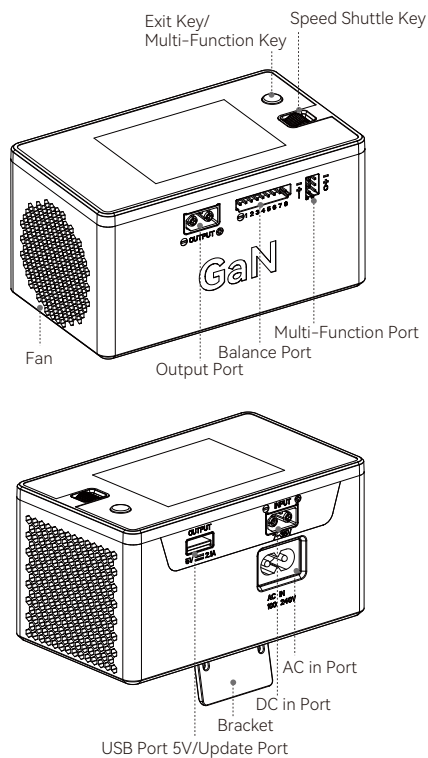
Abbildungen der Anschlüsse und Bedienelemente aus der Originalanleitung.
